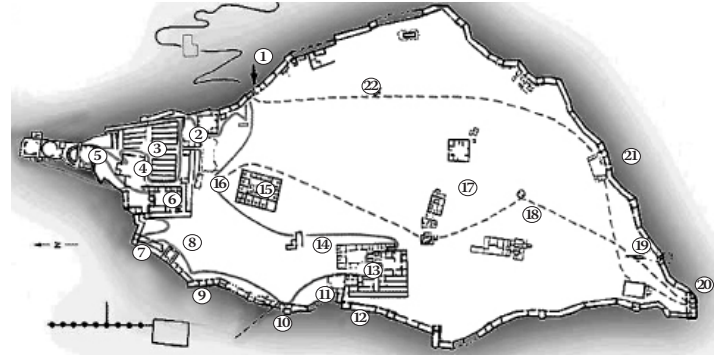
Masada. Plan twierdzy: 1. wejście od ścieżki wężowej; 2. pomieszczenia z łóżkami; 3. magazyny; 4. łaźnie; 5. pałac północny; 6. budynki administracyjne; 7. punkt obserwacyjny; 8. synagoga; 9. mur kazamatowy i biblioteka; 10. rampa rzymska; 11. wejście zachodnie; 12. wieża garbarzy; 13. pałac zachodni; 14. kościółek bizantyjski; 15. dzielnica urzędników; 16. wieża strażnicza; 17. rezydencje; 18. nisza z urnami; 19. wielka cyster-na; 20. twierdza południowa; 21. mury i dom zelotów; 22. bizantyjska cela monastyczna
